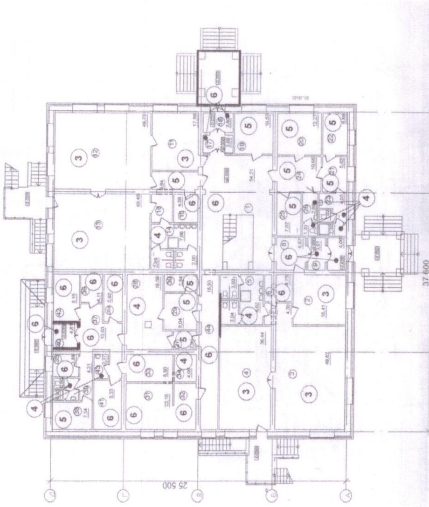
План-схема 1-го этажа
